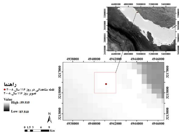
شکل ۵. نقشه مدل سازی شوری قبل از اعتبارسنجی برای روز ۱۶ سال ۲۰۰۸
