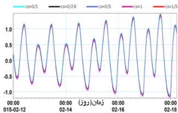
شکل ۳. حساسیت‌سنجی تراز سطح آب نسبت ضریب گرانروی گردابه‌ای
