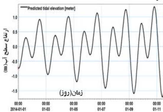
شکل ۴. تغییرات تراز سطح آب اعمال شده به مرز دریا (جداول آدمیرالتی)
