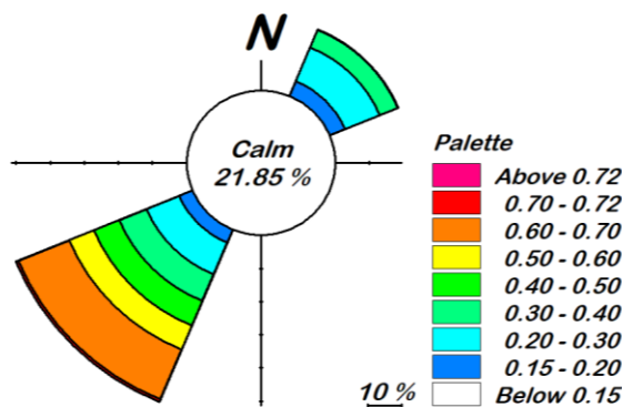
شکل ۱۳. گل جریان در پیچ خسروآباد دبی 480 \text{ m}^3/\text{s}
