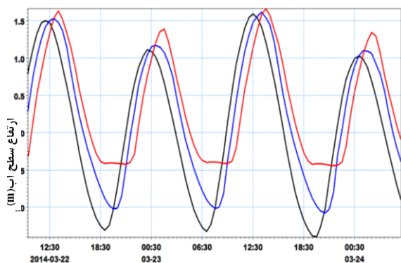
شکل ۷. مقایسه تراز سطح آب در سه ایستگاه مختلف؛ دهانه (سیاه)، فاو (آبی) و پیچ خسروآباد (قرمز)
