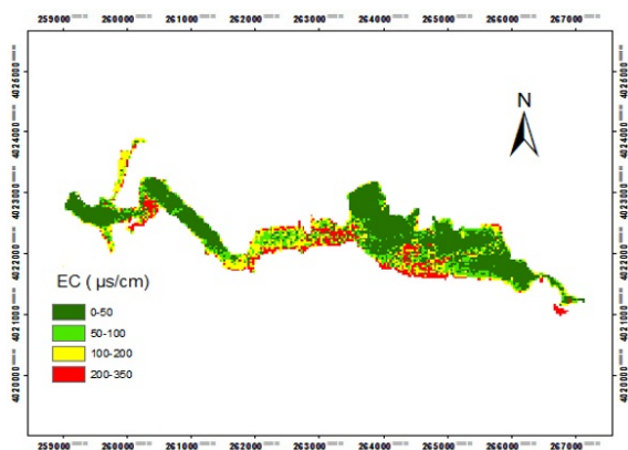
شکل ۱۰. اختلاف دو نقشه توزیع EC به دست آمده با مقادیر مشاهداتی و پیش‌بینی شده مرداد ۱۳۹۴
