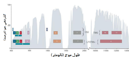
شکل ۲. مقایسه توان تفکیک طیفی سنجنده‌های OLI و TIRS در لندست ۸ و سنجنده ETM+ در لندست ۷
