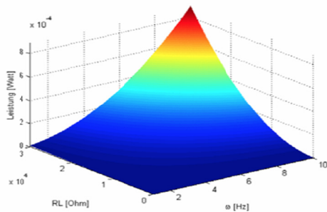
شکل ۱۲. توان خروجی تئوری متوسط حاصل از ژنراتورهای پیزوالکتریکی
