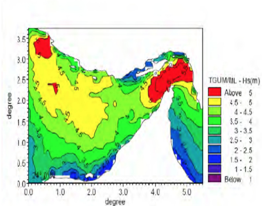
شکل ۶. حداکثر ارتفاع موج در خلیج فارس برای دوره صدساله [۵]
