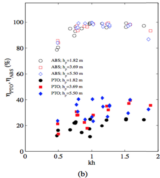
شکل ۵. مقادیر اندازه گیری شده راندمان جذب و PTO برای سه ارتفاع مختلف پمپ ( h_p ) بر حسب kh . شکل a. فرش b1، شکل b2 فرش b2
