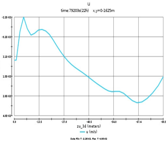
شکل ۱۰: نمایه سرعت افقی u در حالت همرفت آزاد
