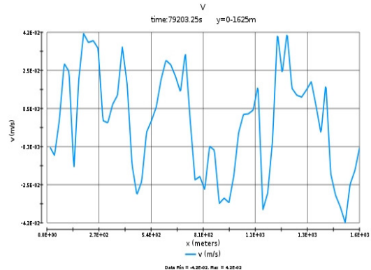
شکل ۱۹: سرعت افقی v در حالت همرفت آزاد
