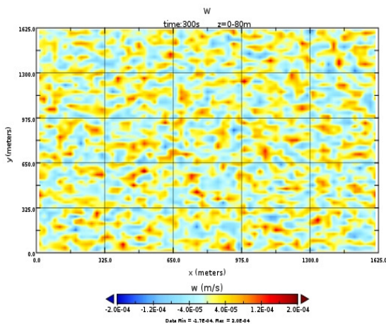
شکل ۱: سطح مقطع سرعت قائم w ، راستای افق در شروع شبیه‌سازی در حالت همرفت آزاد
