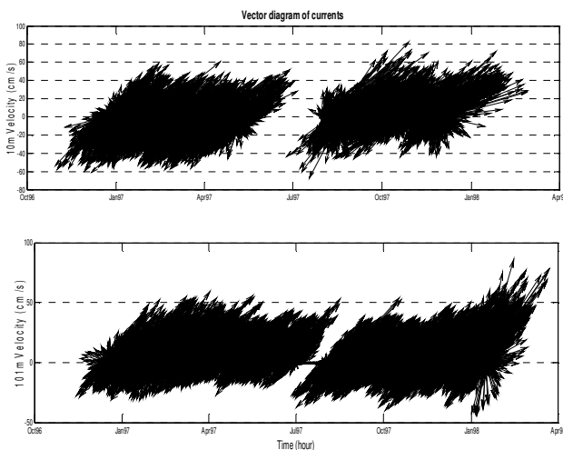
شکل ۲. روند تغییرات زمانی برداری سرعت برای عمق ۱۰ و ۱۰۱ متری.
