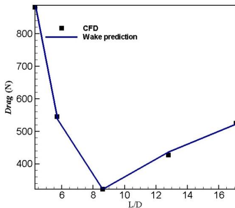
شکل ۱۰. مقایسه نیروی درگ برحسب نسبت منظری از دو روش انتگرال گیری سطح (CFD) و وویک
