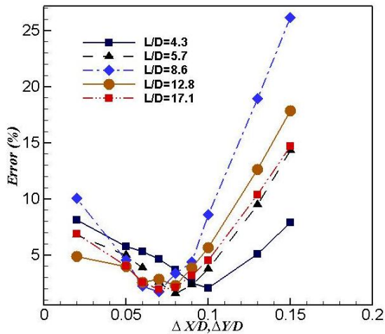
شکل ۹. نحوه تغییرات مقدار متوسط خطا برحسب پارامتری بعد شده اندازه شبکه در نسبت های منظری مختلف
