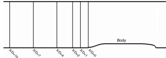
شکل ۱۱. مقاطع مختلف برای استخراج نیروی درگ
