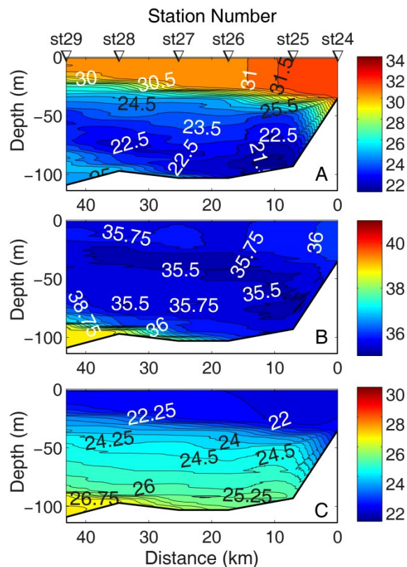
شکل ۹. مشخصات فیزیکی آب در محدوده‌ی شرقی تنگه‌ی هرمز برای فصل تابستان: (A) دمای آب، (B) شوری آب، (C) \sigma_t آب.
