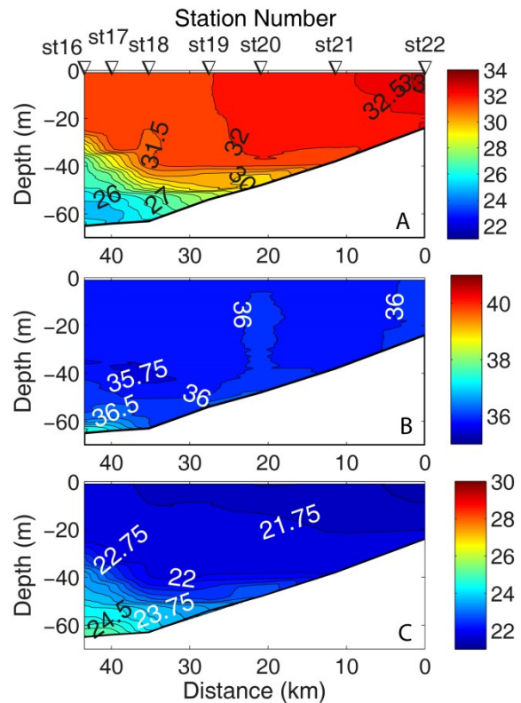
شکل ۸. مشخصات فیزیکی آب در محدوده‌ی مرکزی تنگه‌ی هرمز برای فصل تابستان: (A) دمای آب، (B) شوری آب، (C) \sigma_t آب.
